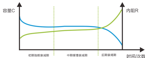
▲ 寿命曲线图
