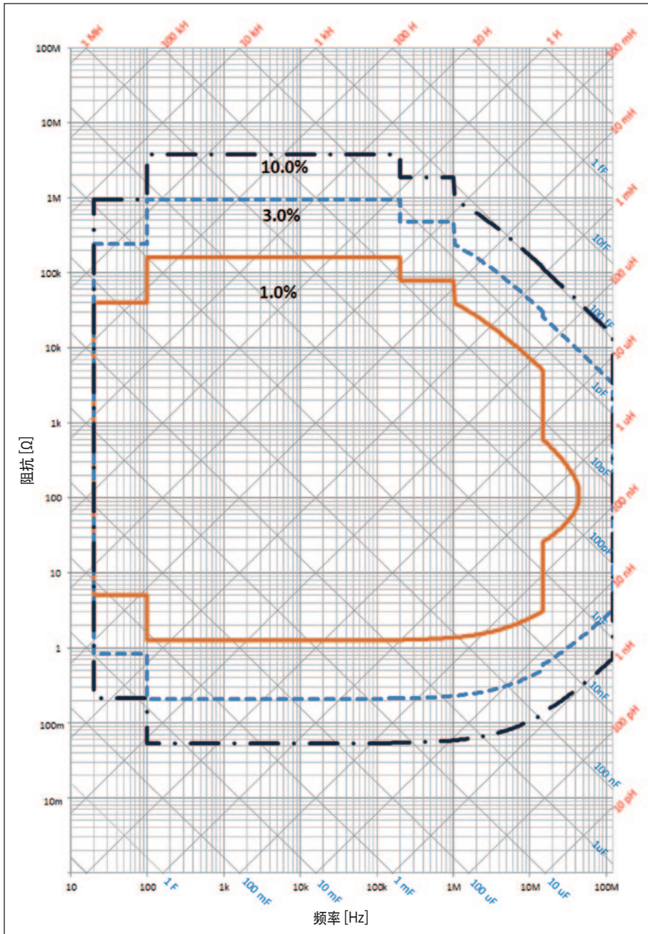
图 6. Keysight 42942A 端适配器连接至 E4990A (振荡器电平 = 0.5 Vrms) 时, 其 7 毫米端口的阻抗测量精度, 测量时间 = 5
