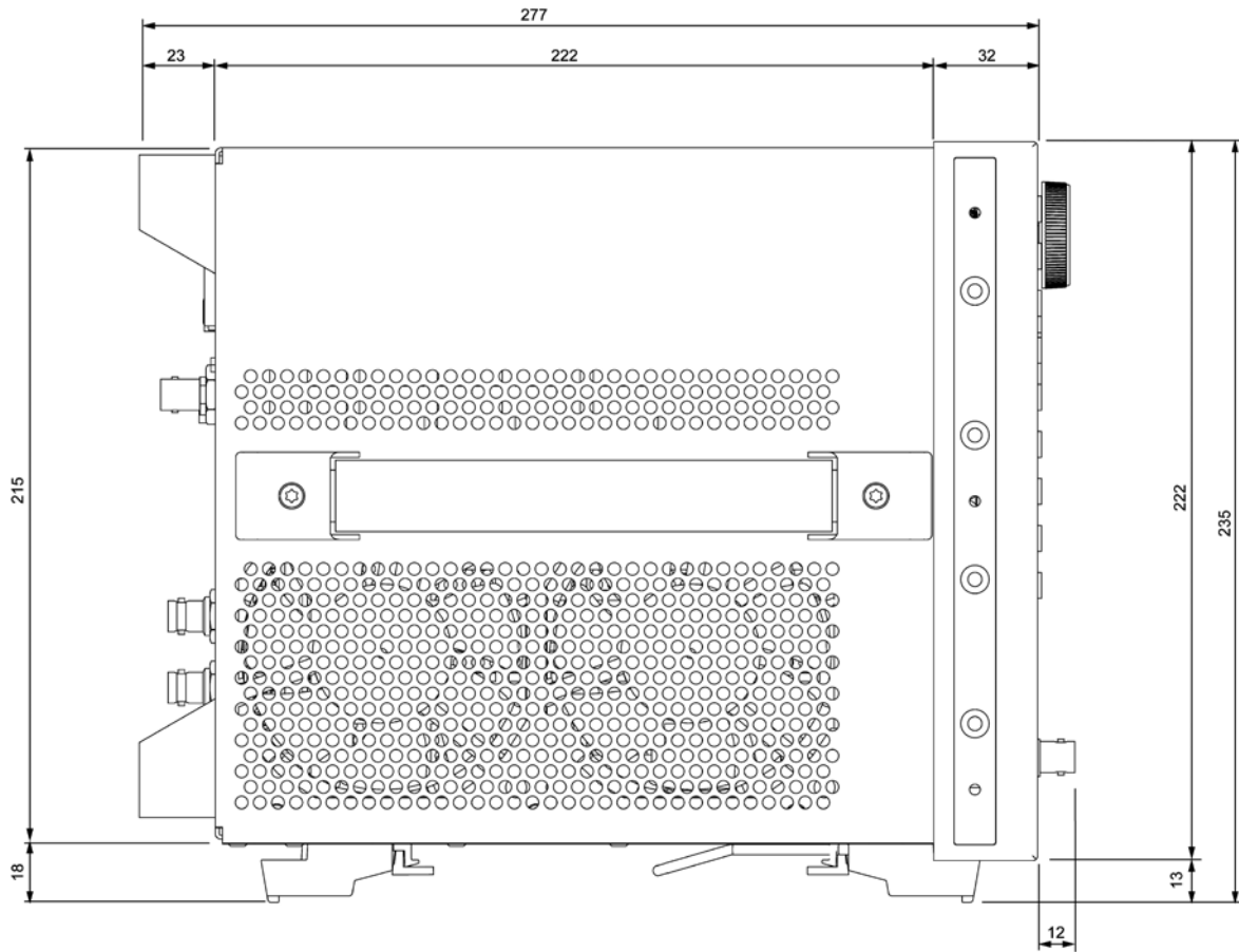
图 12. 侧视图 (毫米)
