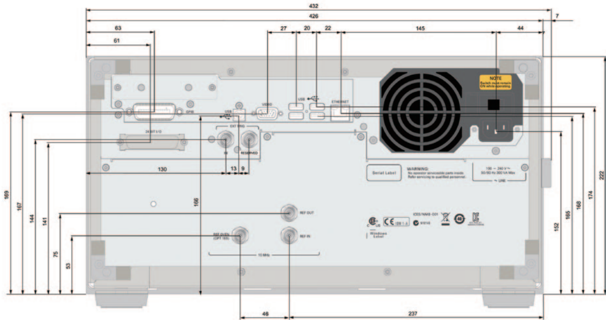
图 11. 后视图(毫米)
