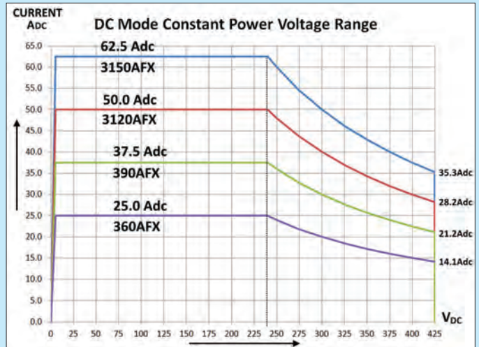
AFX单相直流输出时功率曲线
