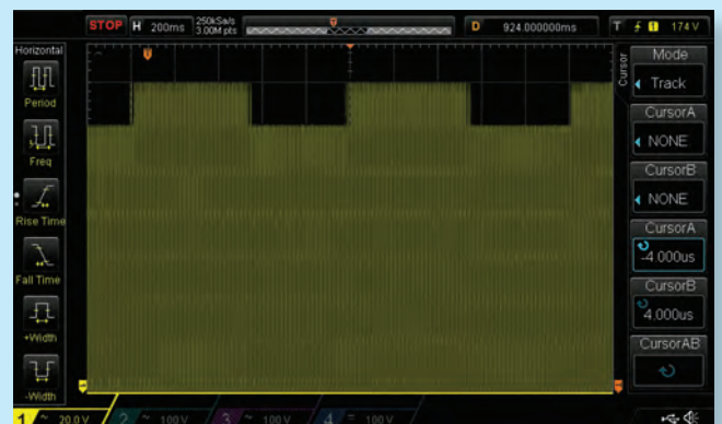
电压调制测试 @ 1Hz
